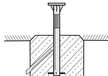
Sockelpfosten für Kabelanschlußkasten
