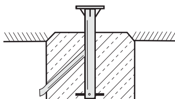
Sockelpfosten mit Kabelführungsrohr
