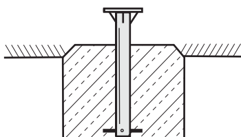
Sockelpfosten zum Einbetonieren
